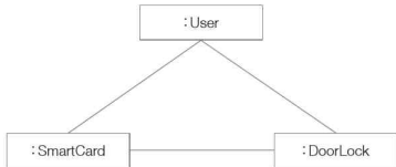
그림 6-5 디지털 도어록의 객체 다이어그램
